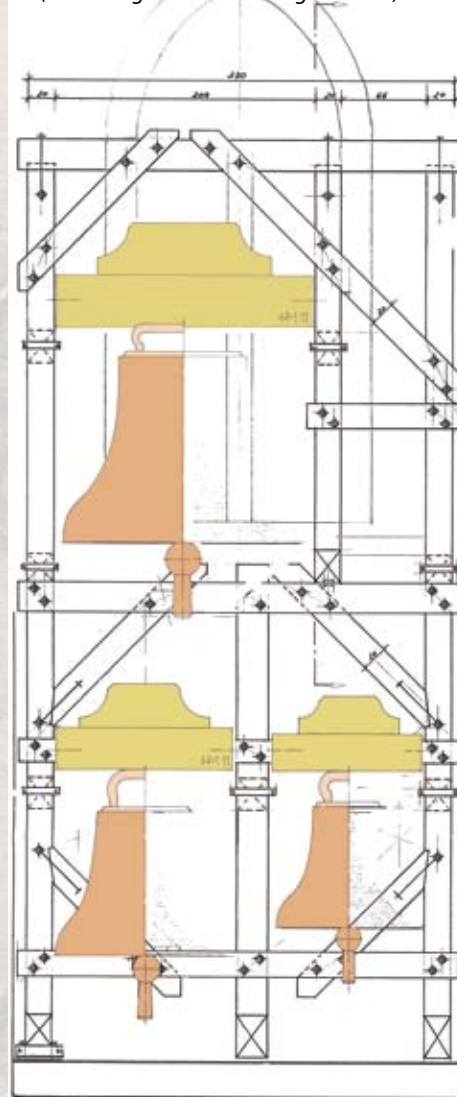
Der Glockenstuhl im Südturm (Zeichnung Metz nach Vorlage Bachert)
